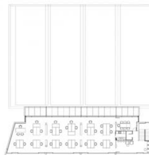
Neckom centar osnova prizemlja (gore), prvog sprata (sredina) i drugog sprata (dolje)
